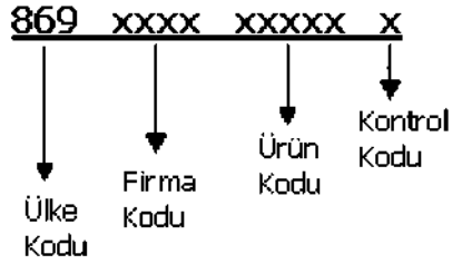
Şekil 1.15: EAN kodlaması
